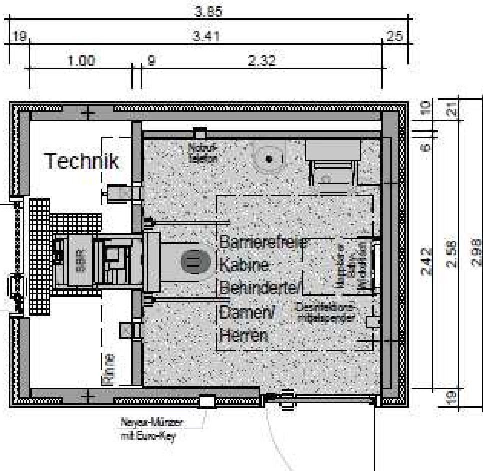
Grundriss
