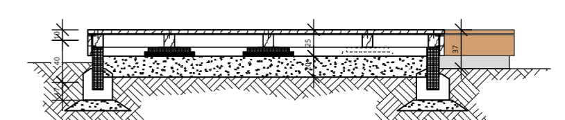
Detail Sitzpodest/Schnitt 1 1:50
