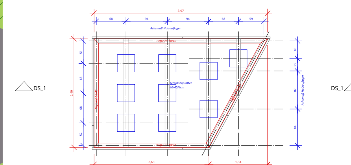
Detail Sitzpodest/Grundriss Auflager 1:50
