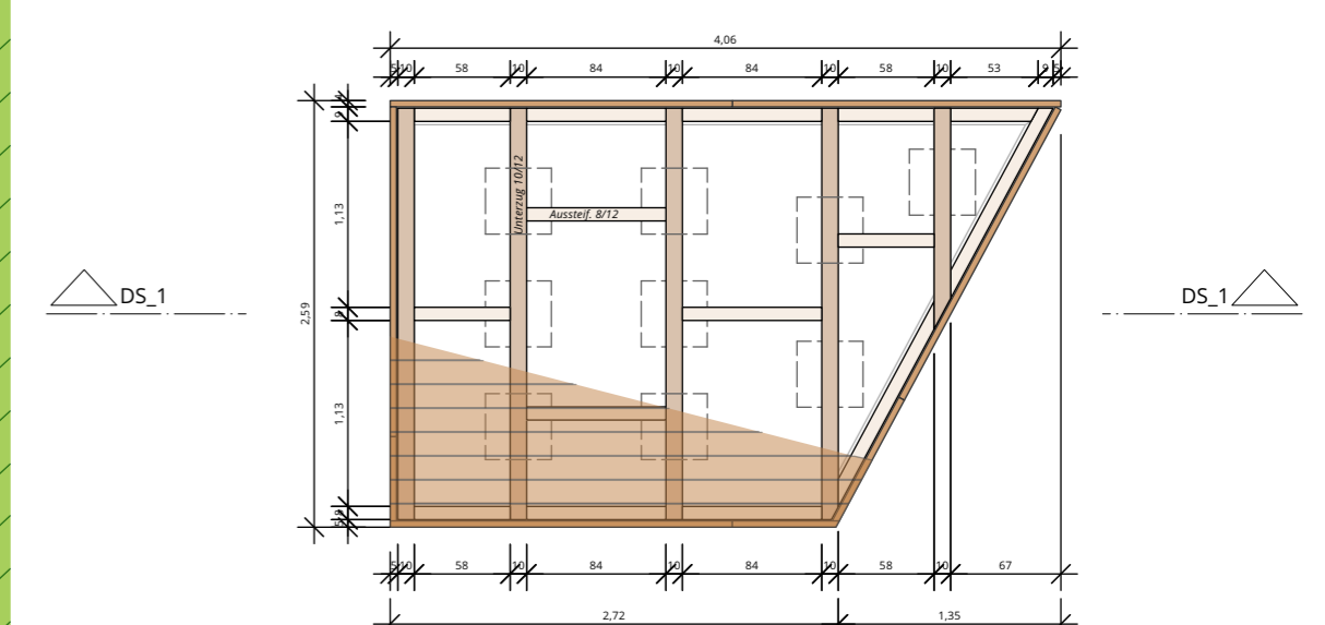
Detail Sitzpodest/Grundriss Unterkonstruktion 1:50
