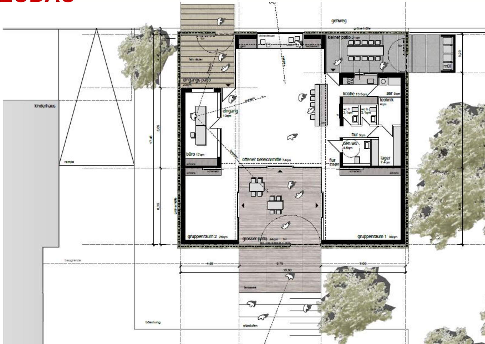
Grundriss Erdgeschoss
